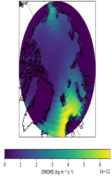
EC-Earth - Arctic - EMIDMS (future_ssp585)
