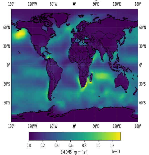
EC-Earth - Global - EMIDMS (future_ssp585)
